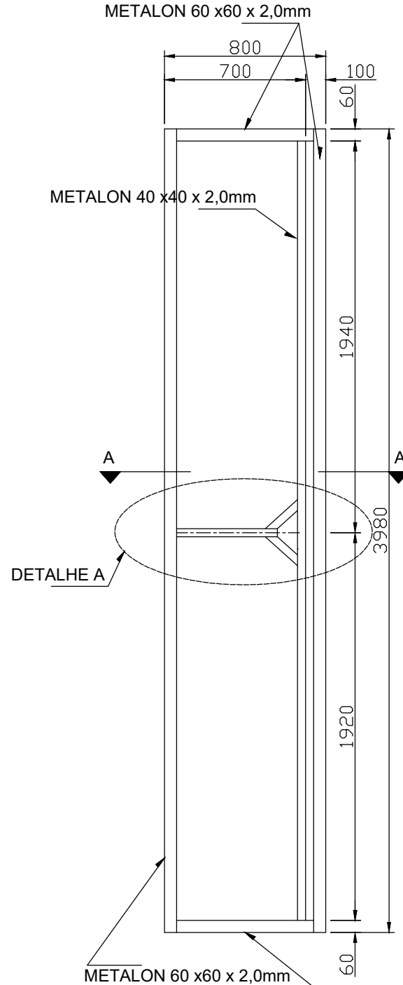
PLATAFORMA SECUNDÁRIA
