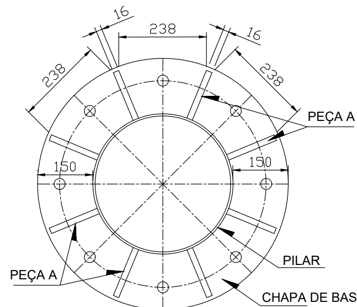
SEÇÃO AA
