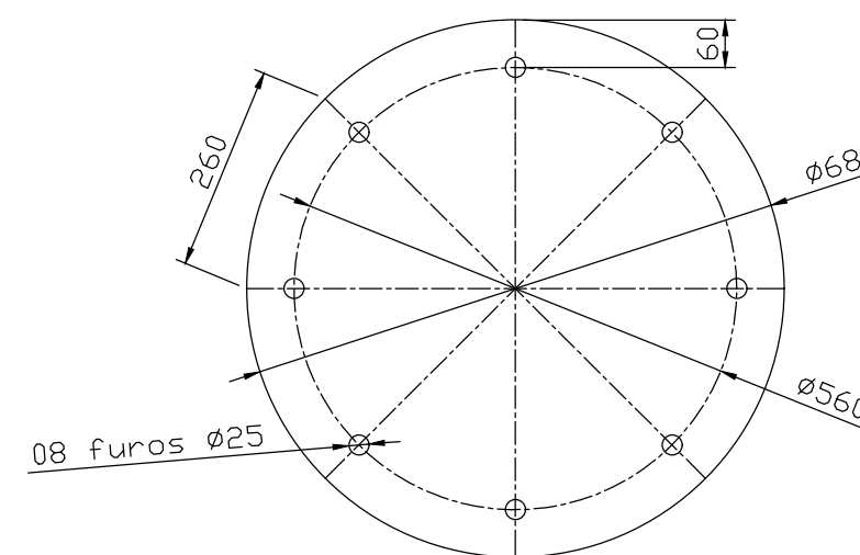
CHAPA GABARITO CHAPA # 14" QUANTIDADE: 01 PÇ
