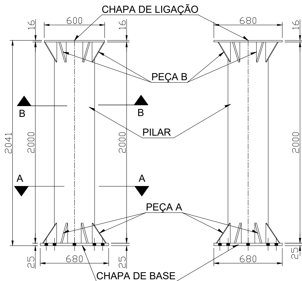
VISTA LATERAL
