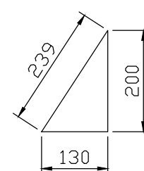
PEÇA B CHAPA # 3/8" QUANTIDADE : 08 PÇS
