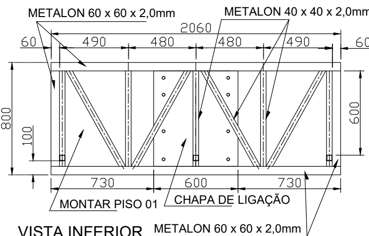
VISTA INFERIOR
