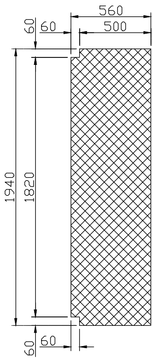
PISO 02 CHAPA EXPANDIDA # 1/8" QUANTIDADE : 01 PÇ
