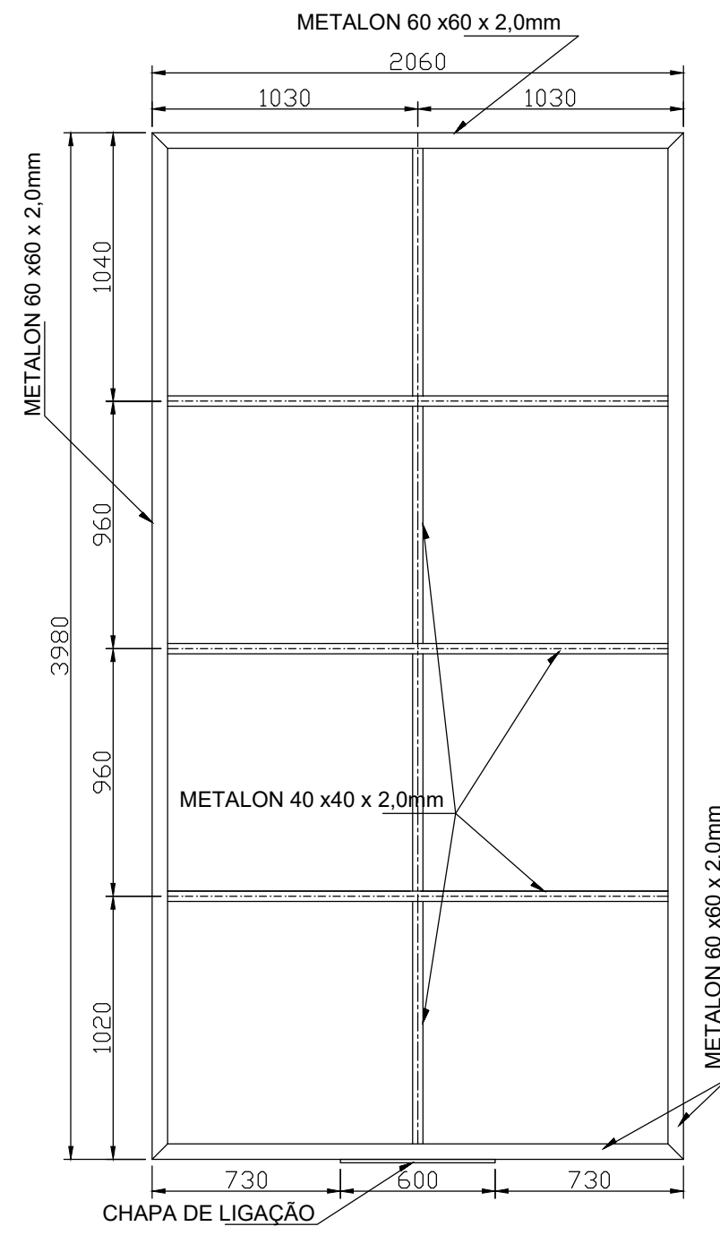
VISTA DO FUNDO
