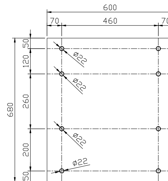
CHAPA DE LIGAÇÃO CHAPA # 5/8" QUANTIDADE: 02 PÇS
