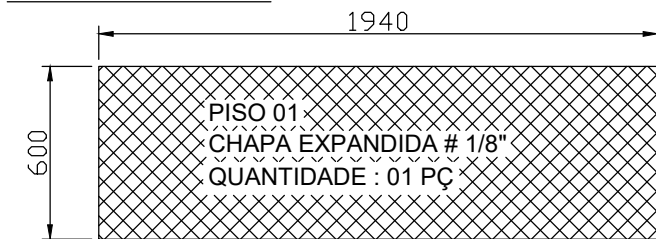
VISTA INFERIOR
