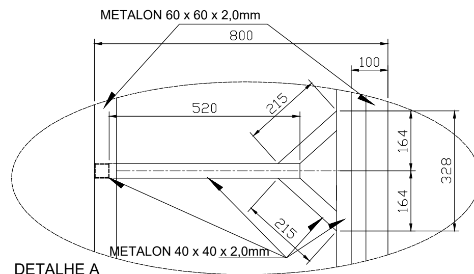
DETALHE A
