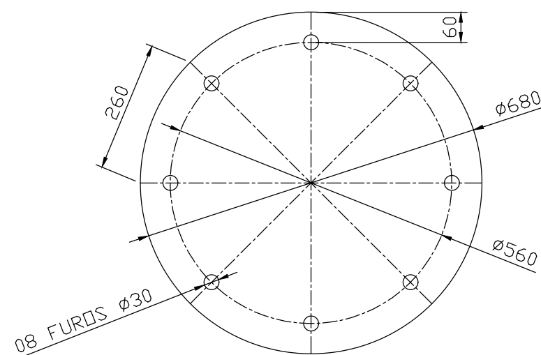
CHAPA DE BASE CHAPA # 1" QUANTIDADE: 01 PÇ
